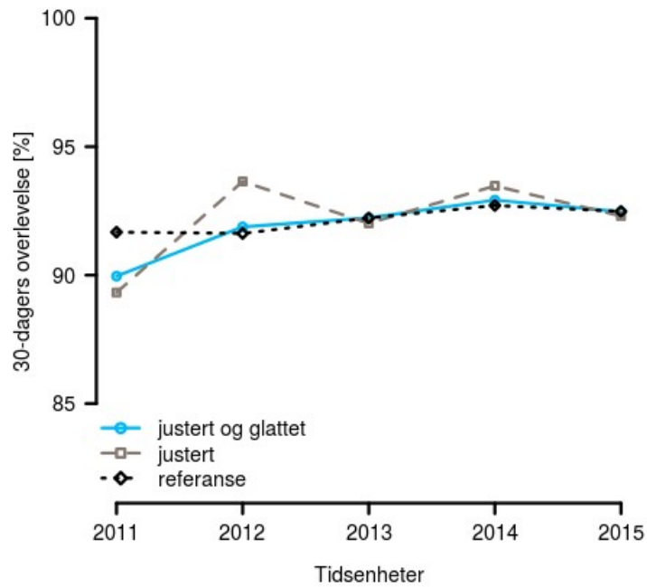
Figur 12 : Tidsutvikling for førstegangs hjerteinfarkt, Levanger (2011-2015)
