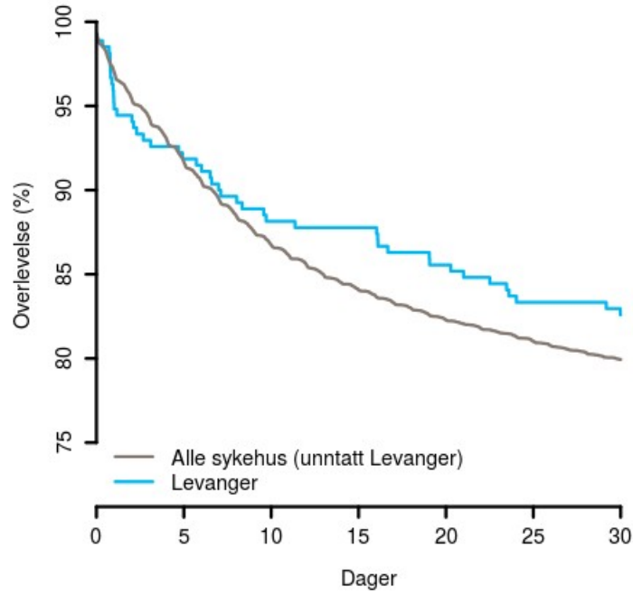
Figur 4 : Kaplan-Meierkurver for hjerneslag, alder > median (75.0 år), Levanger (2013-2015)
