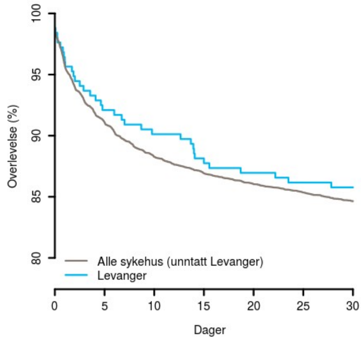
Figur 8 : Kaplan-Meierkurver for førstegangs hjerteinfarkt, alder > median (73.0 år), Levanger (2013-2015)
