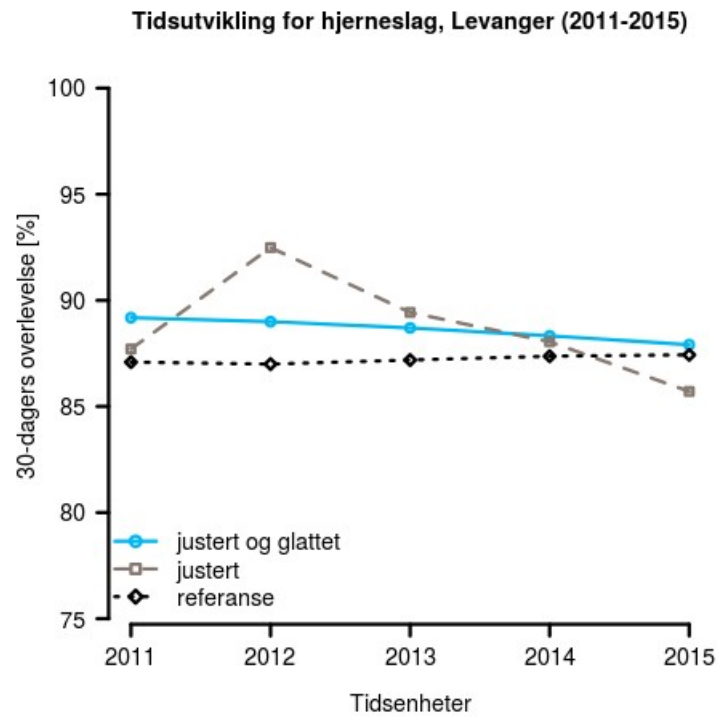
Figur 10 : Tidsutvikling for hjerneslag, Levanger (2011-2015)
