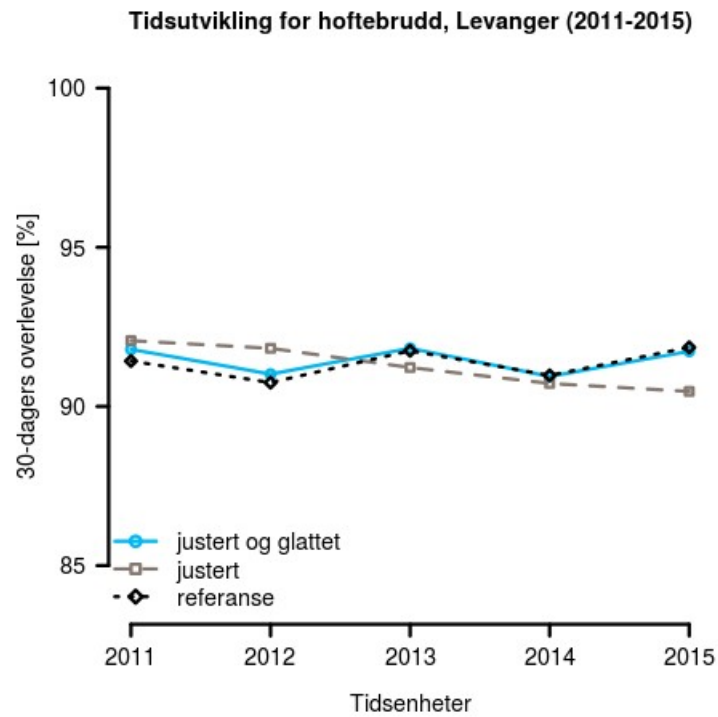
Figur 11 : Tidsutvikling for hoftebrudd, Levanger (2011-2015)
