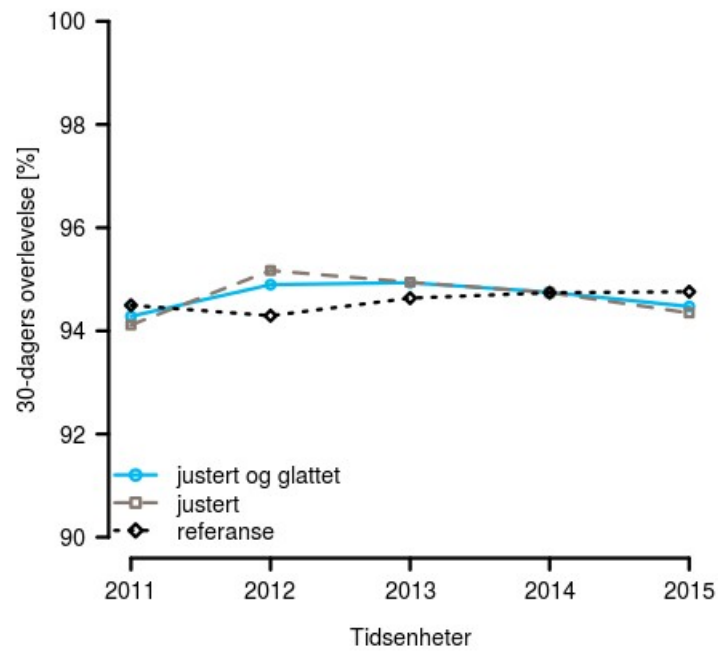
Figur 9 : Tidsutvikling for totaloverlevelse, Levanger (2011-2015)
