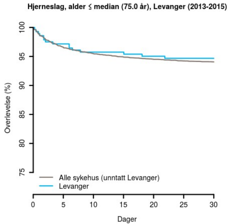
Figur 3 : Kaplan-Meierkurver for hjerneslag, alder \leq median (75.0 år), Levanger (2013-2015)
