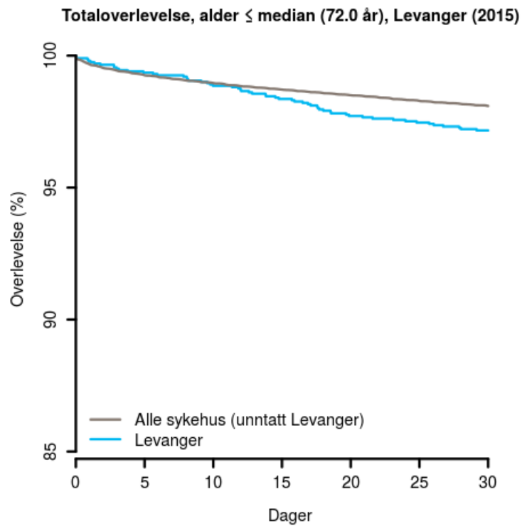
Figur 1 : Kaplan-Meierkurver for totaloverlevelse, alder \leq median (72.0 år), Levanger (2015). Tallene er ikke risikjustert.
