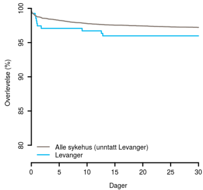
Figur 7 : Kaplan-Meierkurver for førstegangs hjerteinfarkt, alder \leq median (73.0 år), Levanger (2013-2015)
