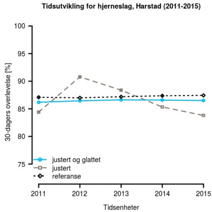
Figur 10 : Tidsutvikling for hjerneslag, Harstad (2011-2015)
