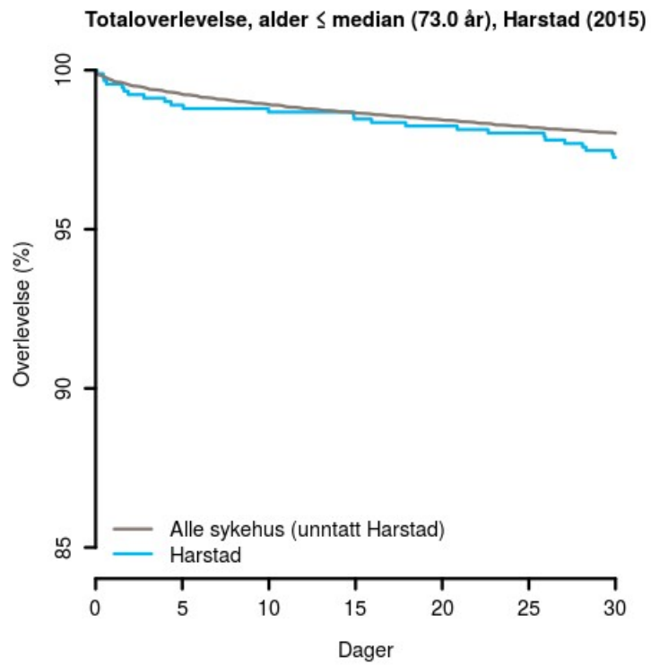
Figur 1 : Kaplan-Meierkurver for totaloverlevelse, alder \leq median (73.0 år), Harstad (2015). Tallene er ikke risikjustert.
