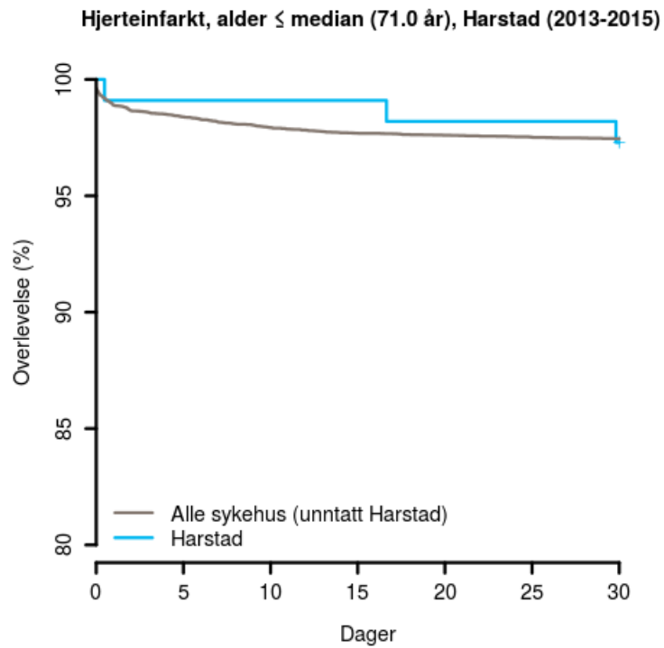
Figur 7 : Kaplan-Meierkurver for førstegangs hjerteinfarkt, alder \leq median (71.0 år), Harstad (2013-2015)
