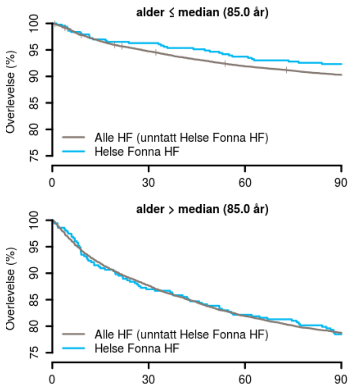
Figur 5 : Kaplan-Meierkurver for hoftebrudd for Helse Fonna HF (2014-2016). Tallene er ikke risikojustert.
