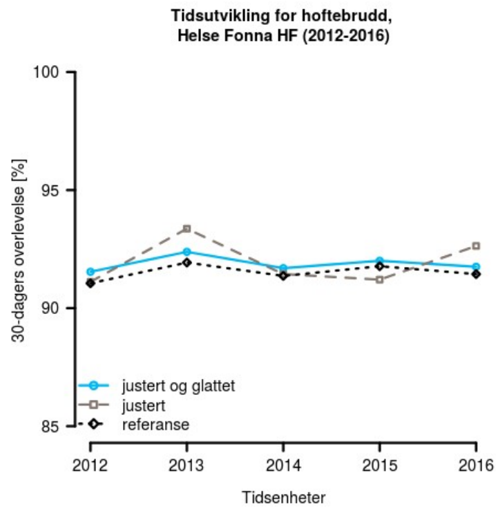
Figur 11 : Tidsutvikling for hoftebrudd, Helse Fonna HF (2012-2016)
