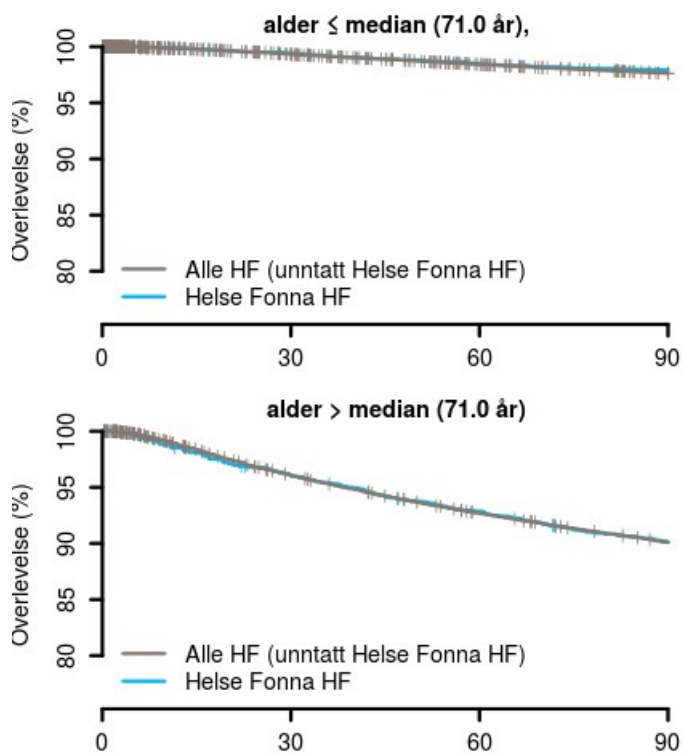
Figur 2 : Kaplan-Meierkurver for totaloverlevelse for pasienter utskrevet som levende for Helse Fonna HF (2016). Tallene er ikke risikojustert.
