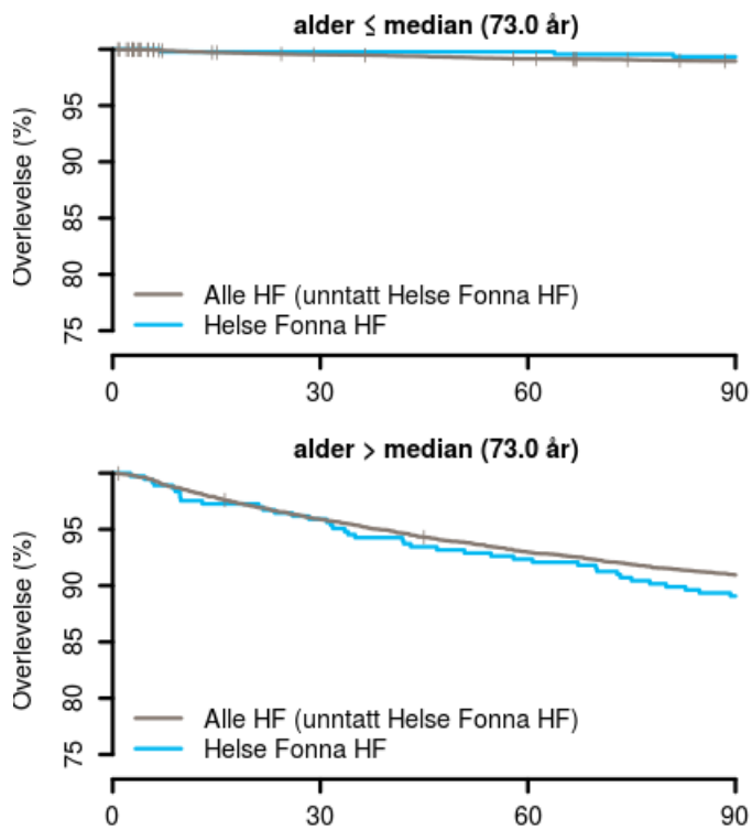
Figur 8 : Kaplan-Meierkurver for førstegangs hjerteinfarkt for pasienter utskrevet som levende for Helse Fonna HF (2014-2016). Tallene er ikke risikjustert.
