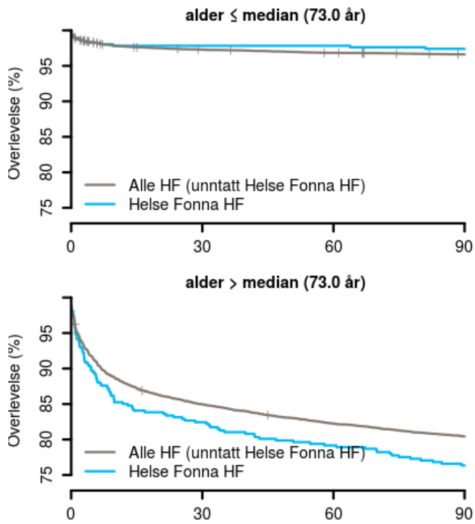
Figur 7 : Kaplan-Meierkurver for førstegangs hjerteinfarkt for Helse Fonna HF (2014-2016). Tallene er ikke risikjustert.
