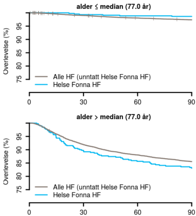
Figur 4 : Kaplan-Meierkurver for hjerneslag for pasienter utskrevet som levende for Helse Fonna HF (2014-2016). Tallene er ikke risikojustert.
