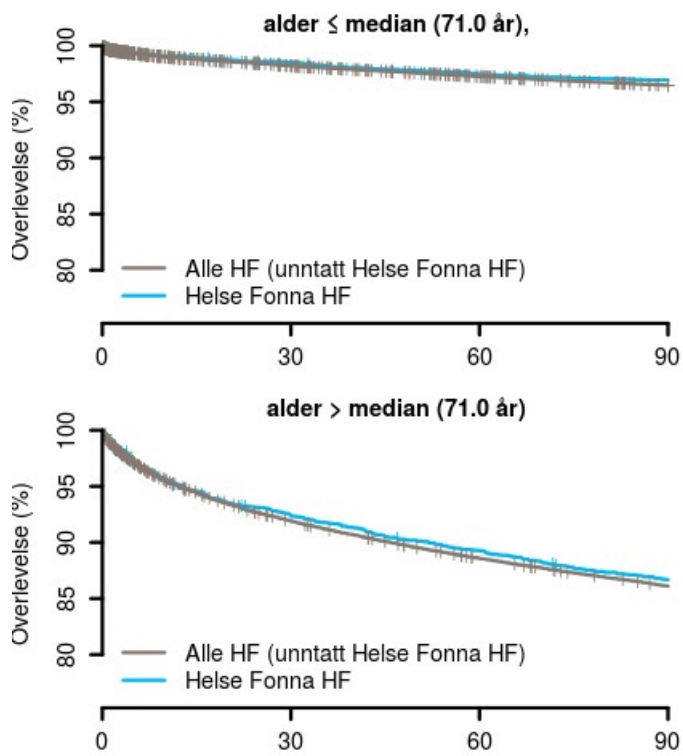
Figur 1 : Kaplan-Meierkurver for totaloverlevelse for Helse Fonna HF (2016). Tallene er ikke risikojustert.
