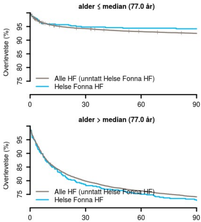
Figur 3 : Kaplan-Meierkurver for hjerneslag for Helse Fonna HF (2014-2016). Tallene er ikke risikojustert.
