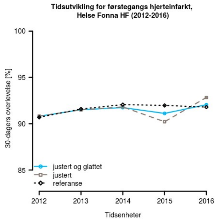
Figur 12 : Tidsutvikling for førstegangs hjerteinfarkt, Helse Fonna HF (2012-2016)
