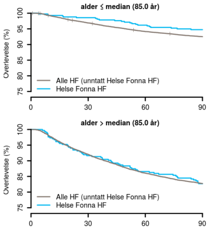
Figur 6 : Kaplan-Meierkurver for hoftebrudd for pasienter utskrevet som levende for Helse Fonna HF (2014-2016). Tallene er ikke risikojustert.
