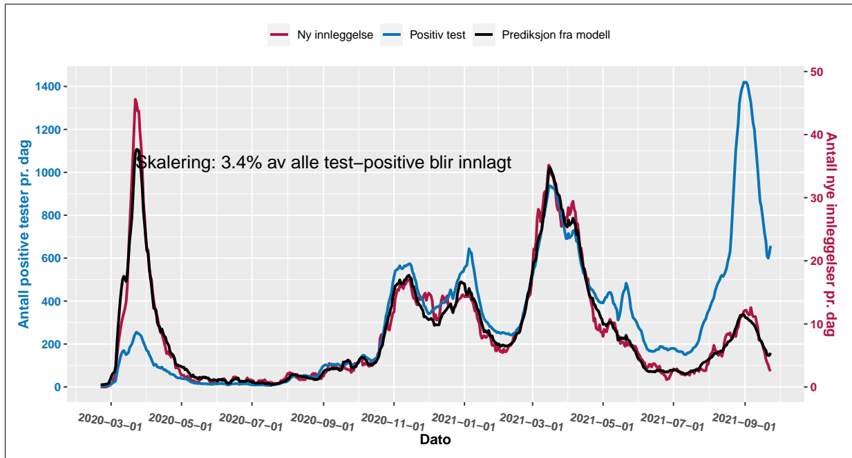
Figur 1: Antall positive tester pr. dag og antall nye innleggelser pr. dag (7 dagers glidende gjennomsnitt) gjennom pandemien. Kurven for innleggelser er skalert og svakt forskjøvet for å lettere kunne sammenlignes med smittetallskurven. Svart kurve viser forventet antall innleggelser, modellestimert fra observerte smittetall.
