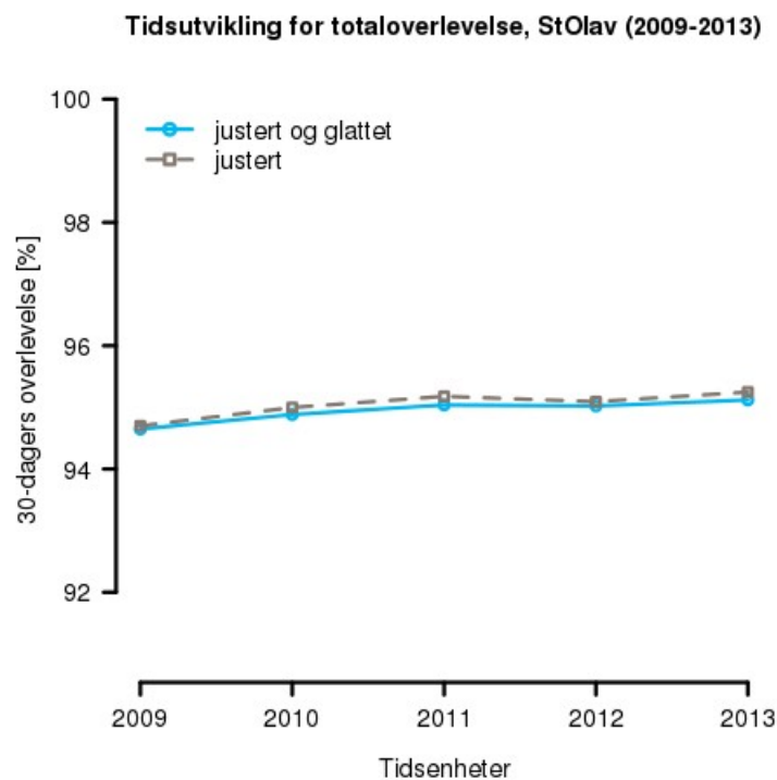
Figur 9 : Tidsutvikling for totaloverlevelse, StOlav (2009-2013)
