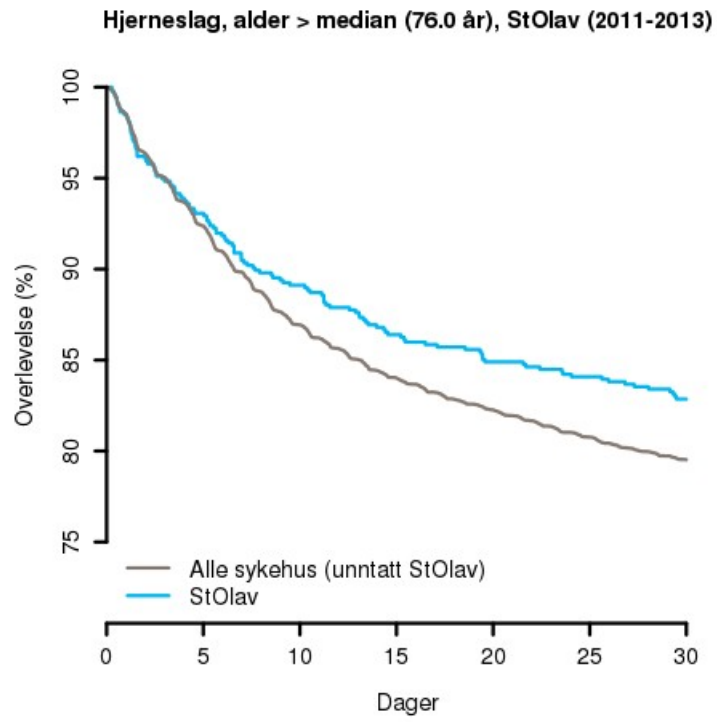
Figur 4 : Kaplan-Meierkurver for hjerneslag, alder > median (76.0 år), StOlav (2011-2013)
