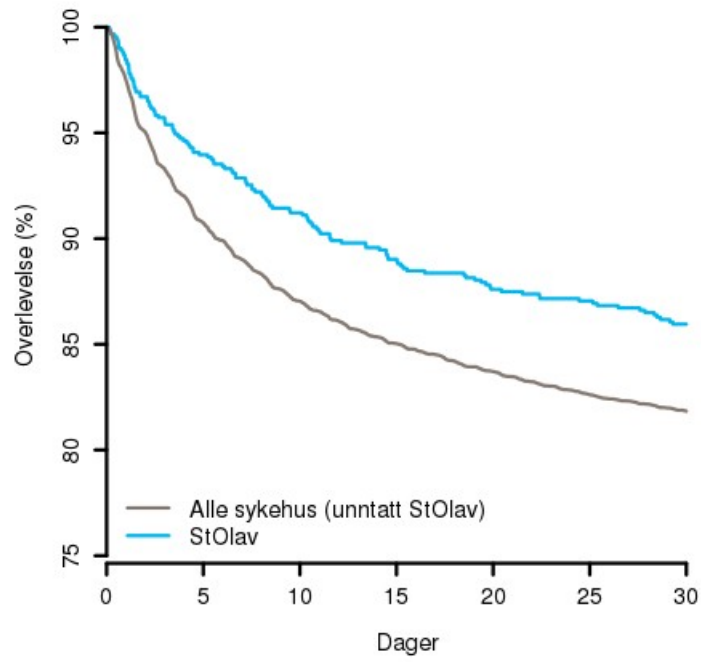
Figur 8 : Kaplan-Meierkurver for førstegangs hjerteinfarkt, alder > median (69.0 år), StOlav (2011-2013)
