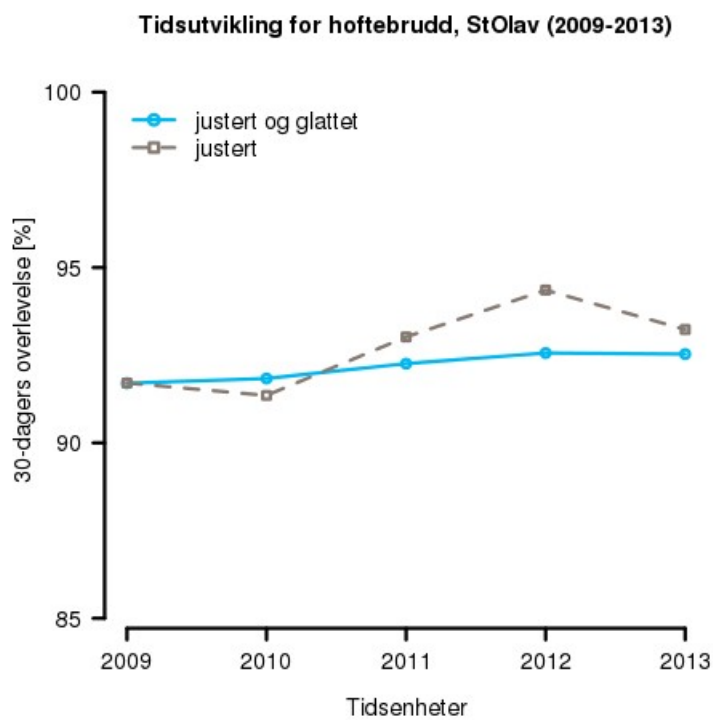
Figur 11 : Tidsutvikling for hoftebrudd, StOlav (2009-2013)
