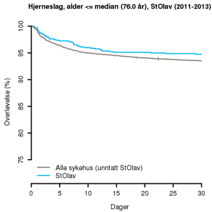
Figur 3 : Kaplan-Meierkurver for hjerneslag, alder <= median (76.0 år), StOlav (2011-2013)
