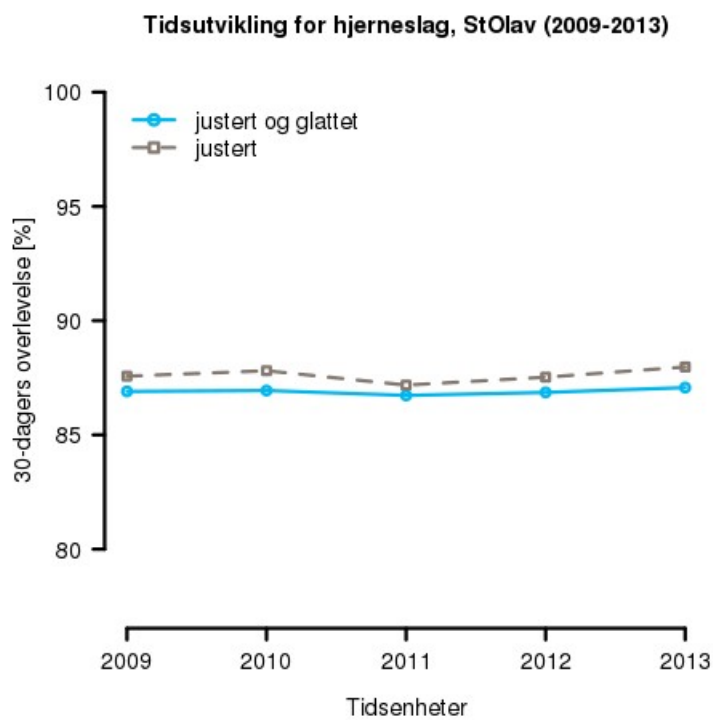
Figur 10 : Tidsutvikling for hjerneslag, StOlav (2009-2013)
