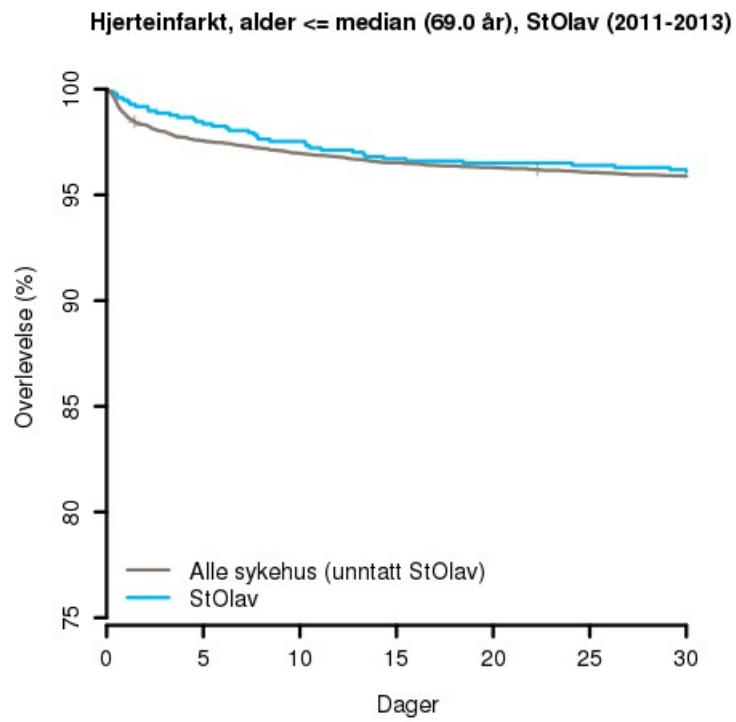
Figur 7 : Kaplan-Meierkurver for førstegangs hjerteinfarkt, alder \leq median (69.0 år), StOlav (2011-2013)
