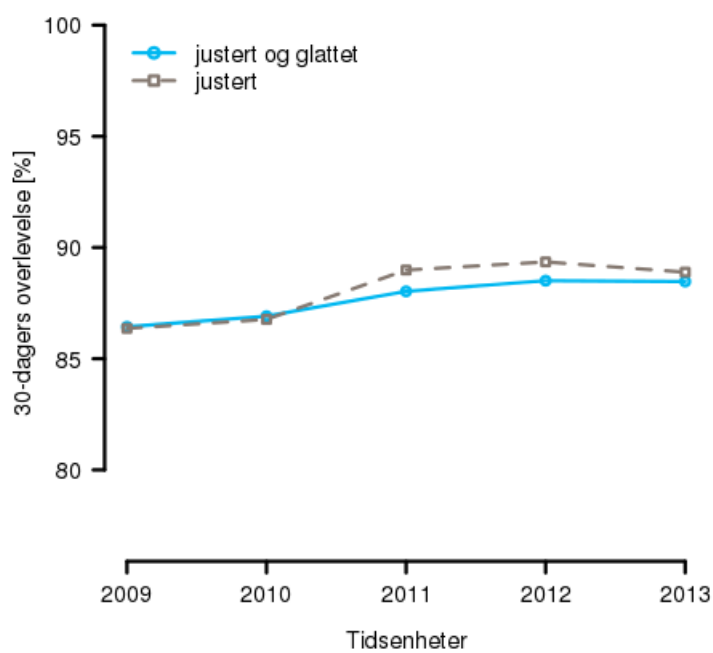
Figur 12 : Tidsutvikling for førstegangs hjerteinfarkt, StOlav (2009-2013)
