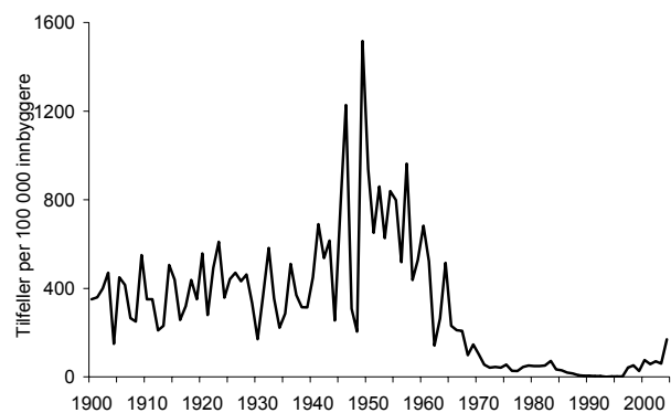
Figur 11. Tilfeller av kikhoste per 100 000 innbyggere i Norge 1900-2004. Kilde: Statistisk sentralbyrå (1900-74) og MSIS (1975-2004).
